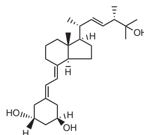
Paricalcitol (Zempar)
