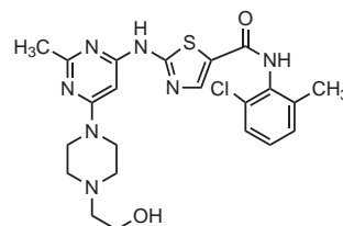
Dasatinib (Sprycel)
