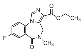
Flumazenil
