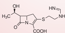
Imipenem
