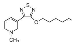
Xanomeline
