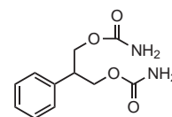
Felbamate
