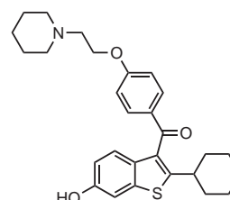
TZE-5323
