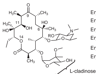
Erythromycin A
